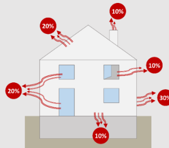
typische Wärmeverluste über die Gebäudehülle [eigene Darstellung]
